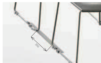
Barra distanziatrice per file - Row distance holder bar
